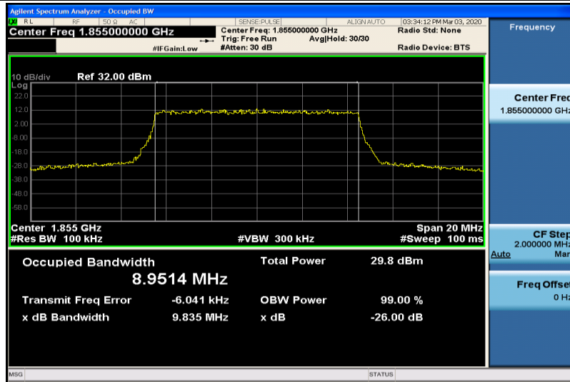
Band2-10MHz-QPSK-18650-50RB#0-8.9514
