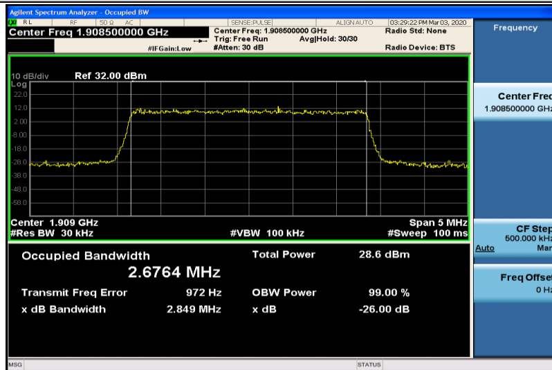
Band2-3MHz-QPSK-19185-15RB#0-2.6764
