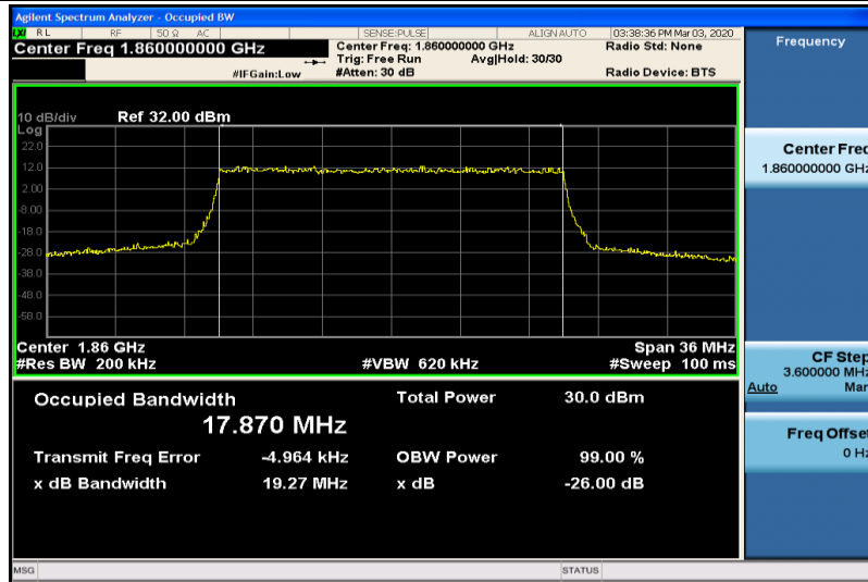
Band2-20MHz-QPSK-18700-100RB#0-17.870
