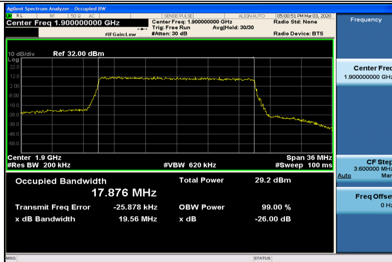
Band2-20MHz-QPSK-19100-100RB#0-17.876
