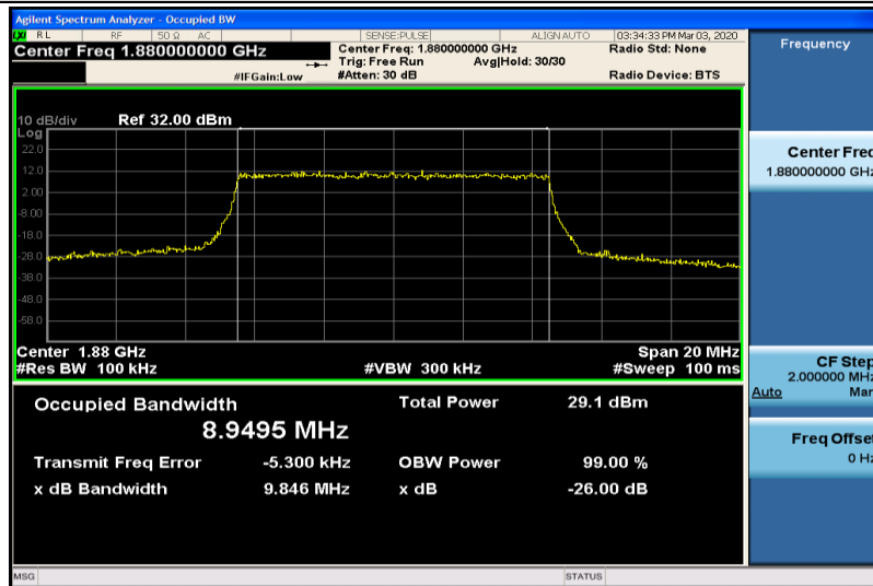
Band2-10MHz-QPSK-18900-50RB#0-8.9495
