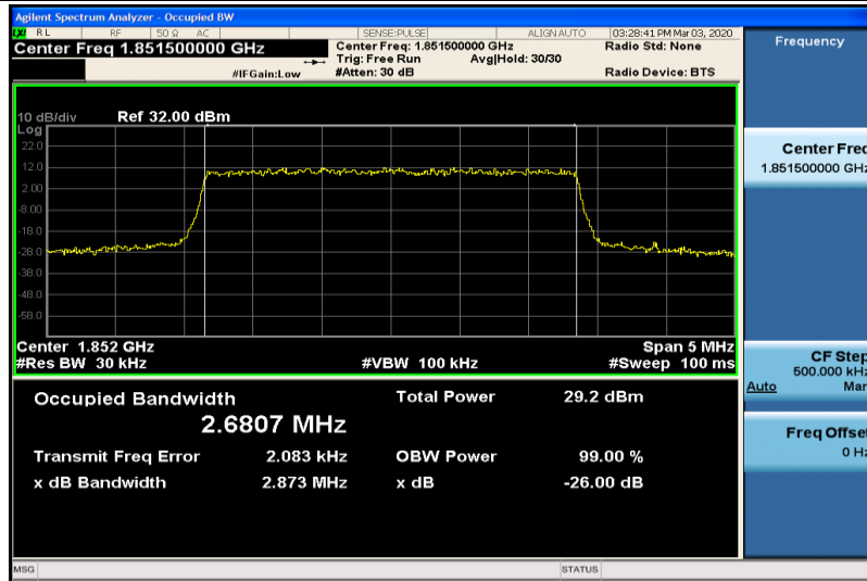
Band2-3MHz-QPSK-18615-15RB#0-2.6807
