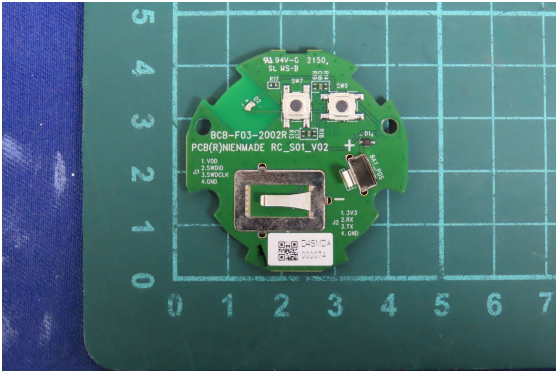
(5) EUT Photo
