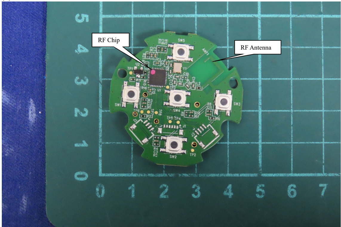
(6) EUT Photo
