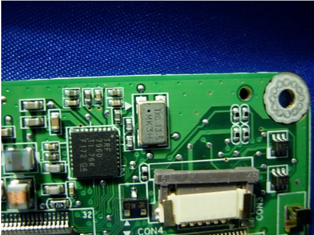
(12) EUT Photo - (RFID Module)
