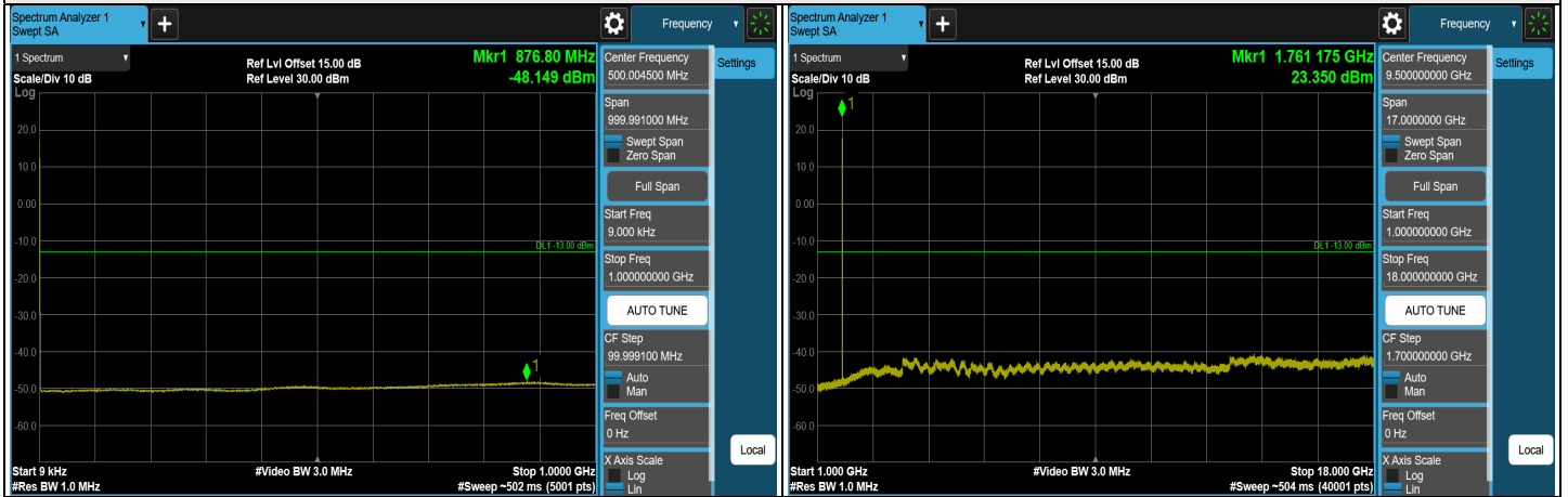
CH 132572 (1770 MHz)
