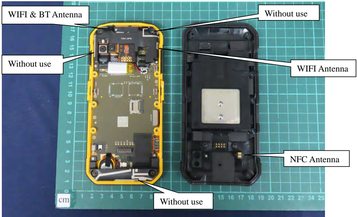
(5) EUT Photo
