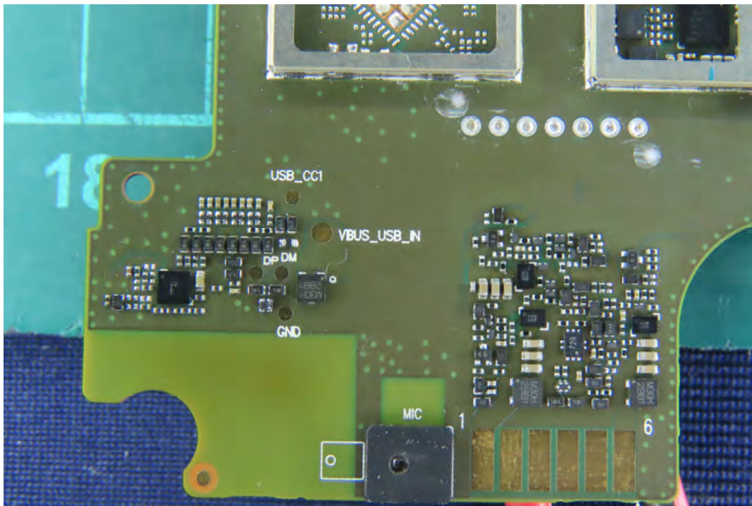
(30) EUT Photo
