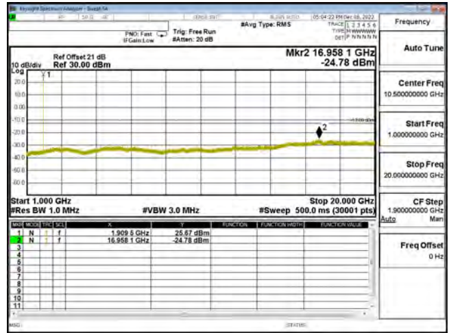
CSE 2G1900 CH810 EGPRS 1G-20G
