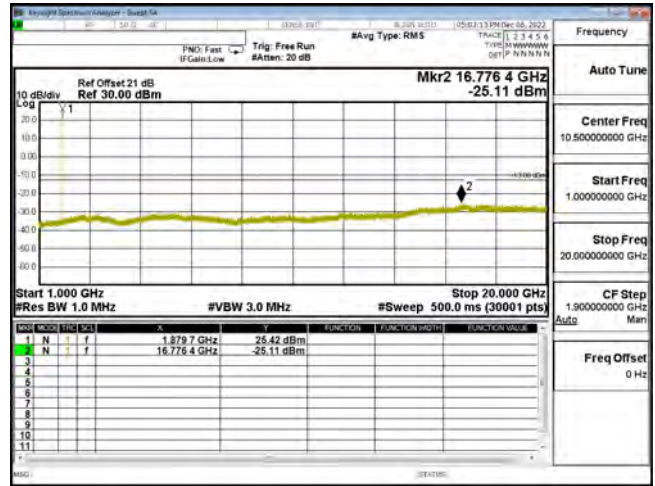
CSE 2G1900 CH661 EGPRS 1G-20G
