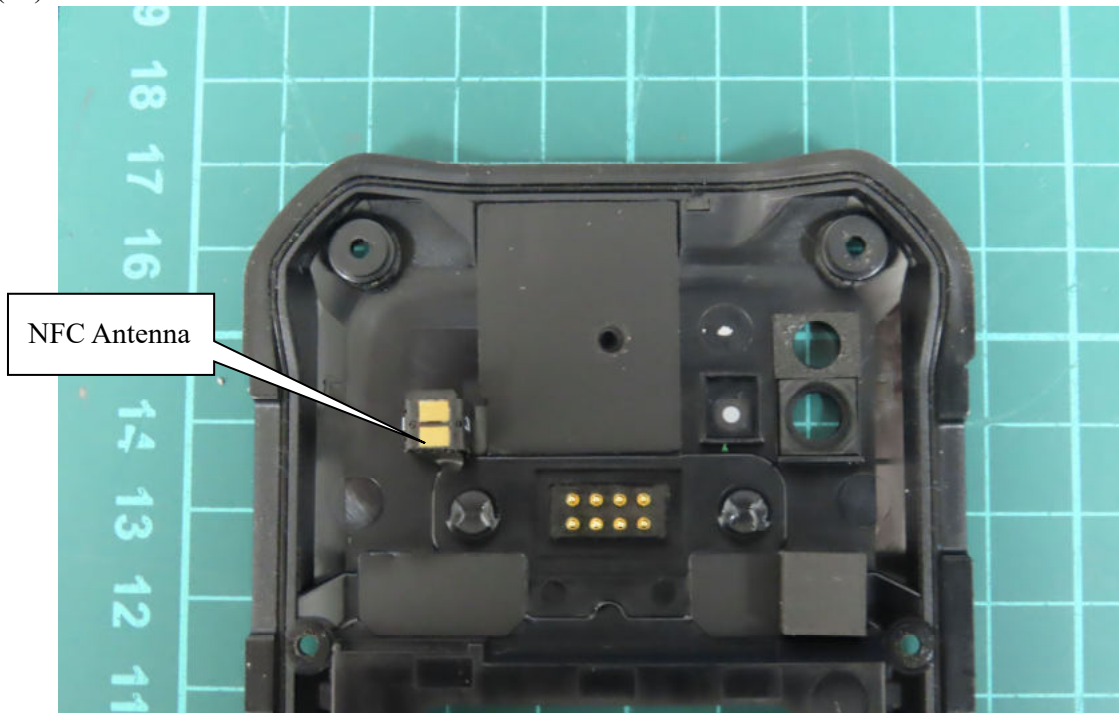
(13) EUT Photo
