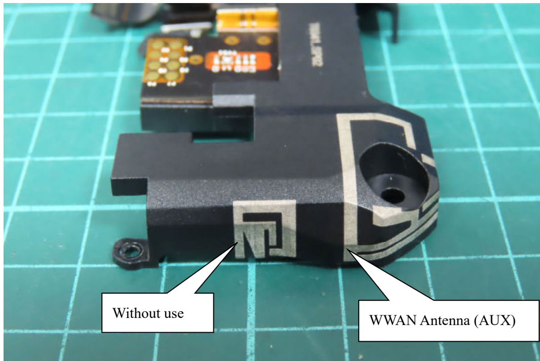
(19) EUT Photo
