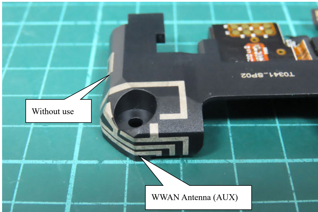
(20) EUT Photo
