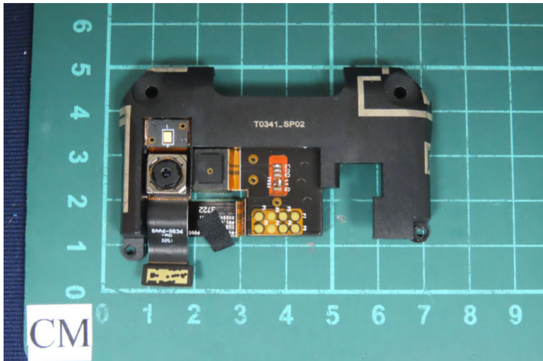
(18) EUT Photo
