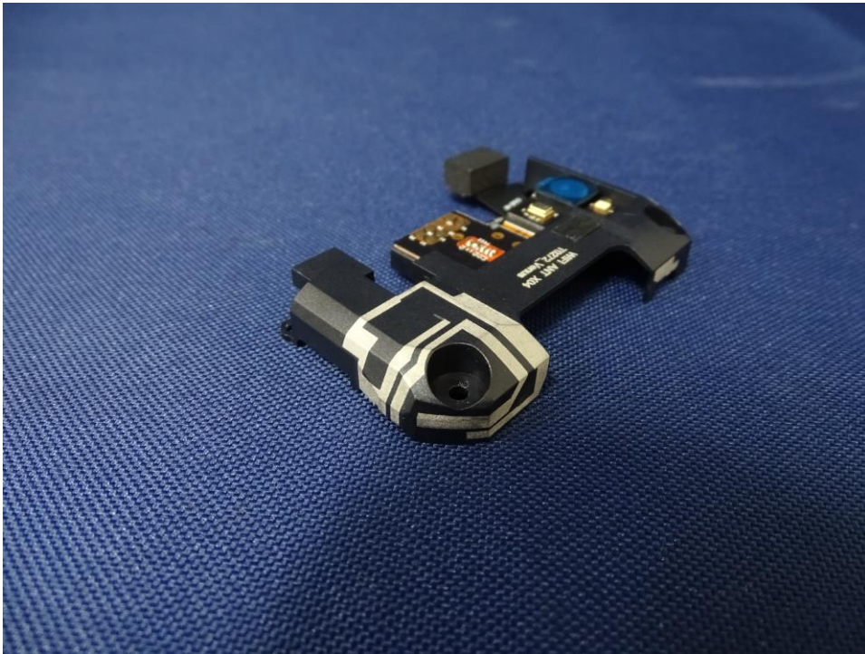
(18) EUT Photo - GPS&WLAN Antenna
