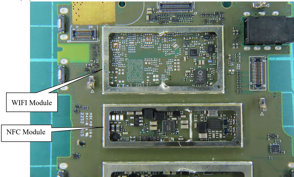
(41) EUT Photo
