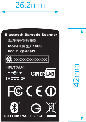
銘版尺寸
