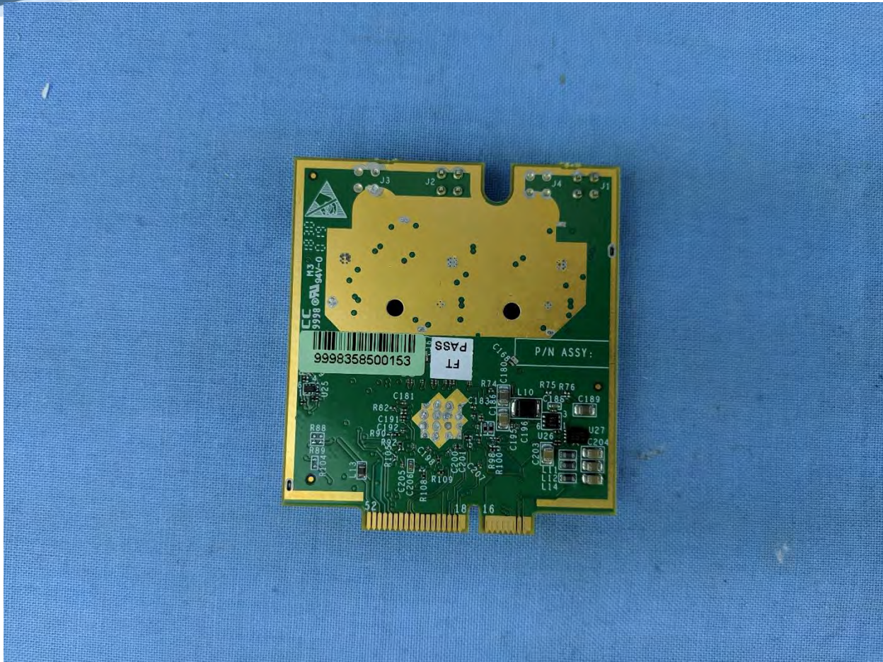
RF Module 1 Back
