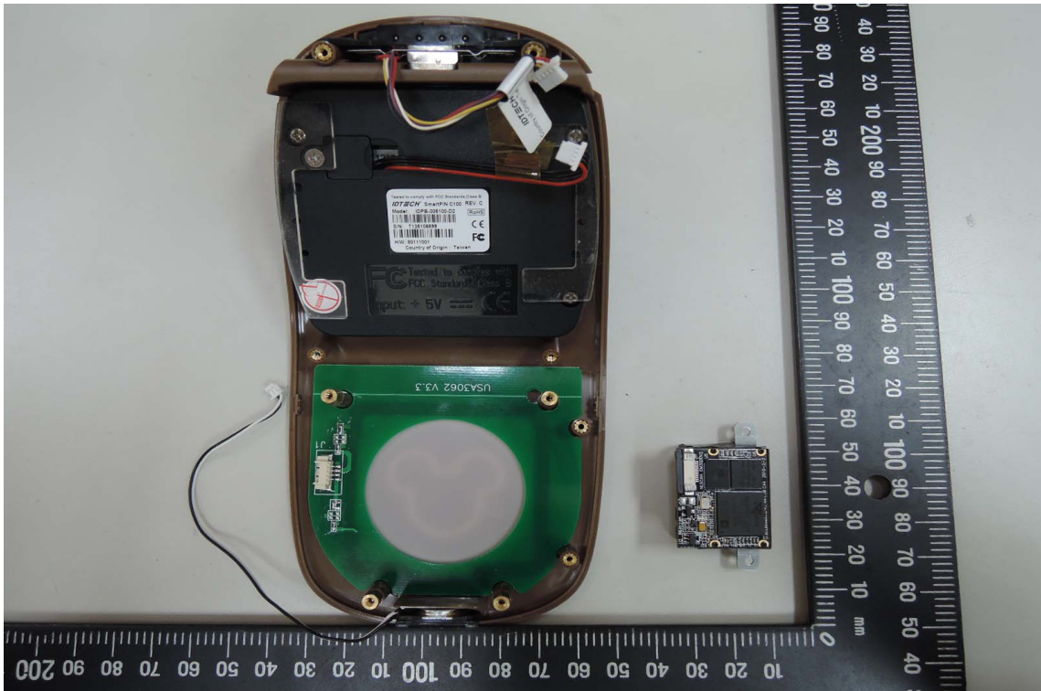
RFID Antenna
