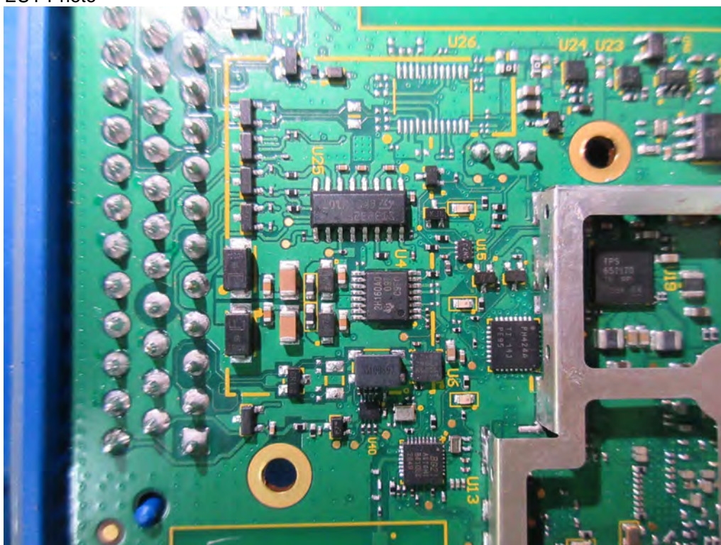
(20) EUT Photo
