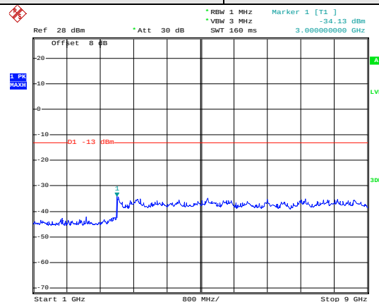
1GHz~9GHz
