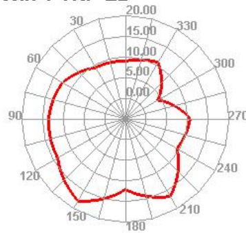
Wifi 1 TRP E2
