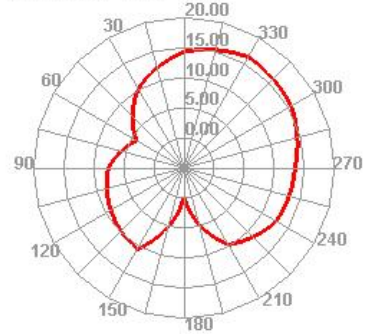
Wifi 165 TRP E2
