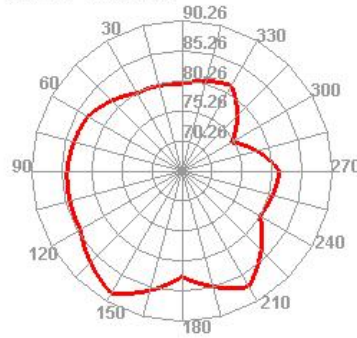
Wifi 1 TIS E2
