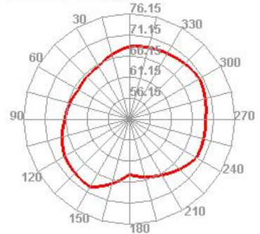
Wifi 36 TIS E2
