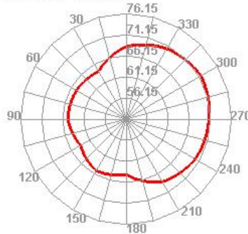
Wifi 36 TIS E1
