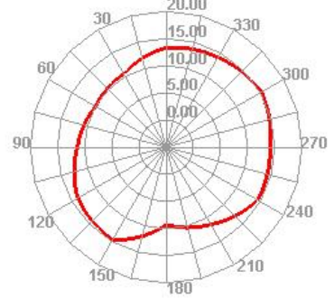
Wifi 36 TRP E2
