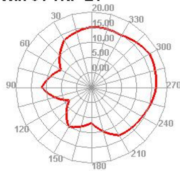
Wifi 64 TRP E1
