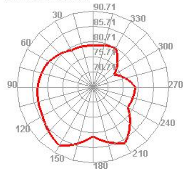
Wifi 6 TIS E2
