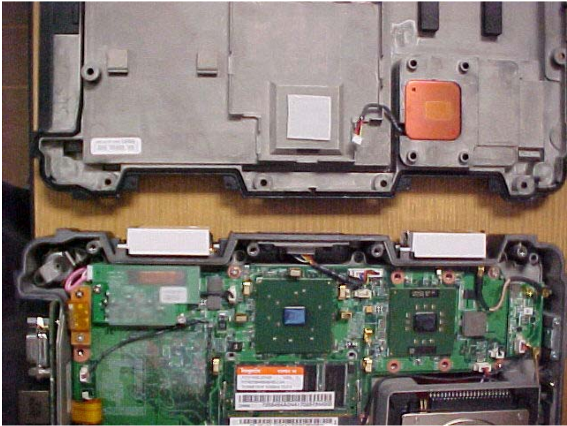
VC-013F – PCB
