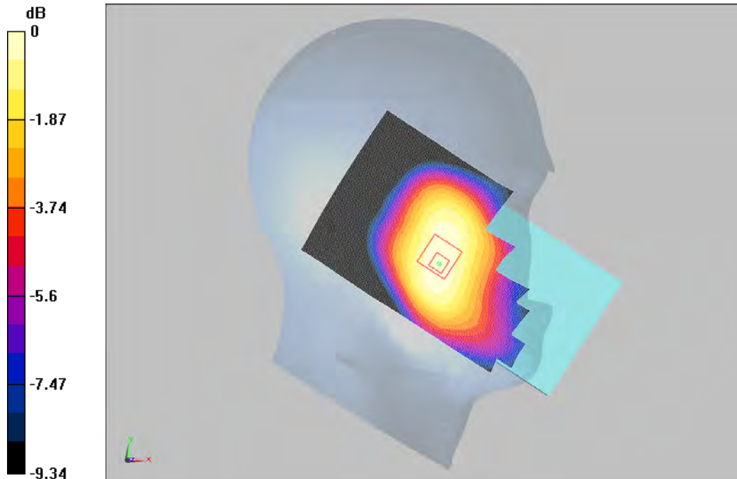
0 dB = 0.197W/kg
