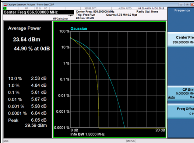
5MHz / 16QAM
