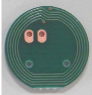
M18 Antenna
