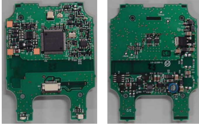
PCB_Main
