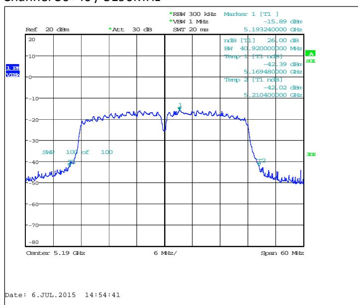
Channel 36+40 / 5190MHz
