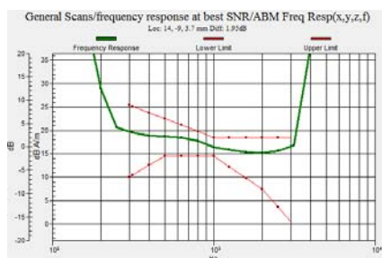
WCDMA1700/2100
