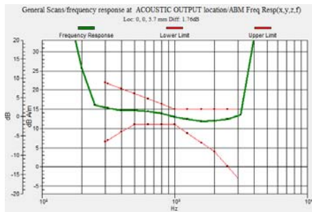
GSM850
