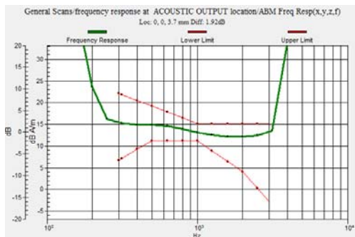
WCDMA850
