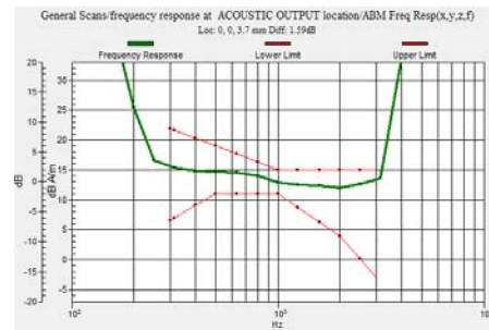
GSM1900
