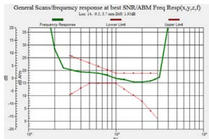
GSM850
