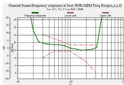
WCDMA1900
