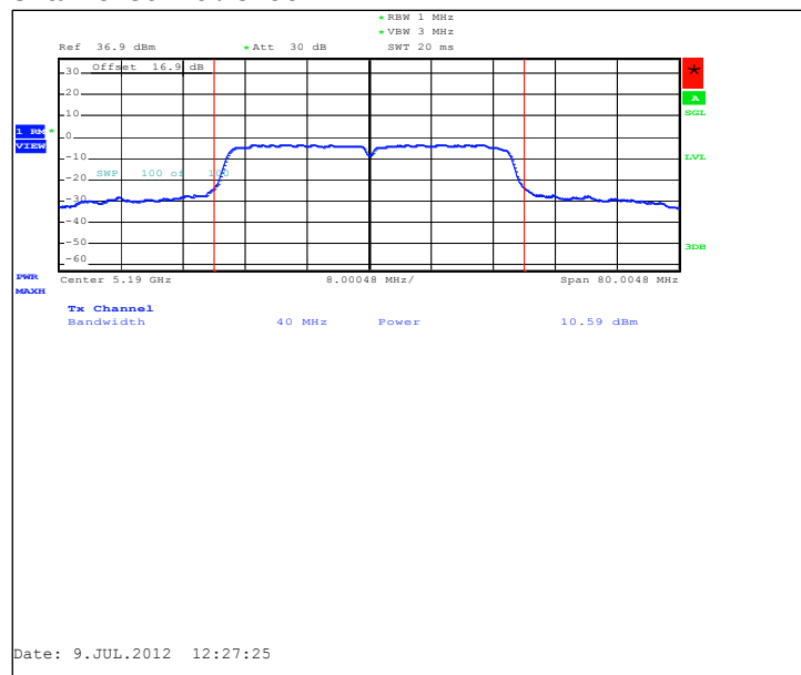
Channel 36+40 / 5190MHz
