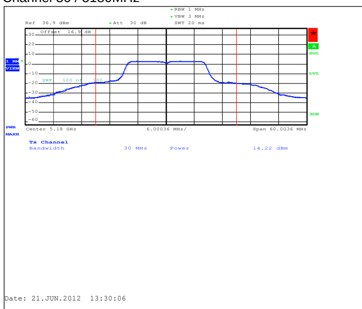
Channel 36 / 5180MHz
