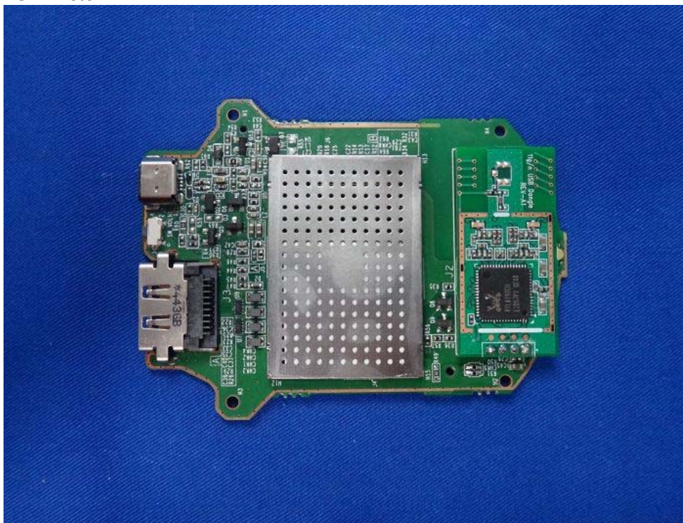
(14) EUT Photo
