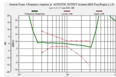
WCDMA1900
