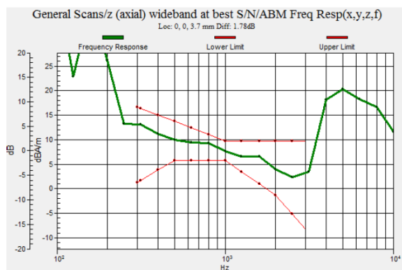
Fig 7.1 GSM850 Ch189
