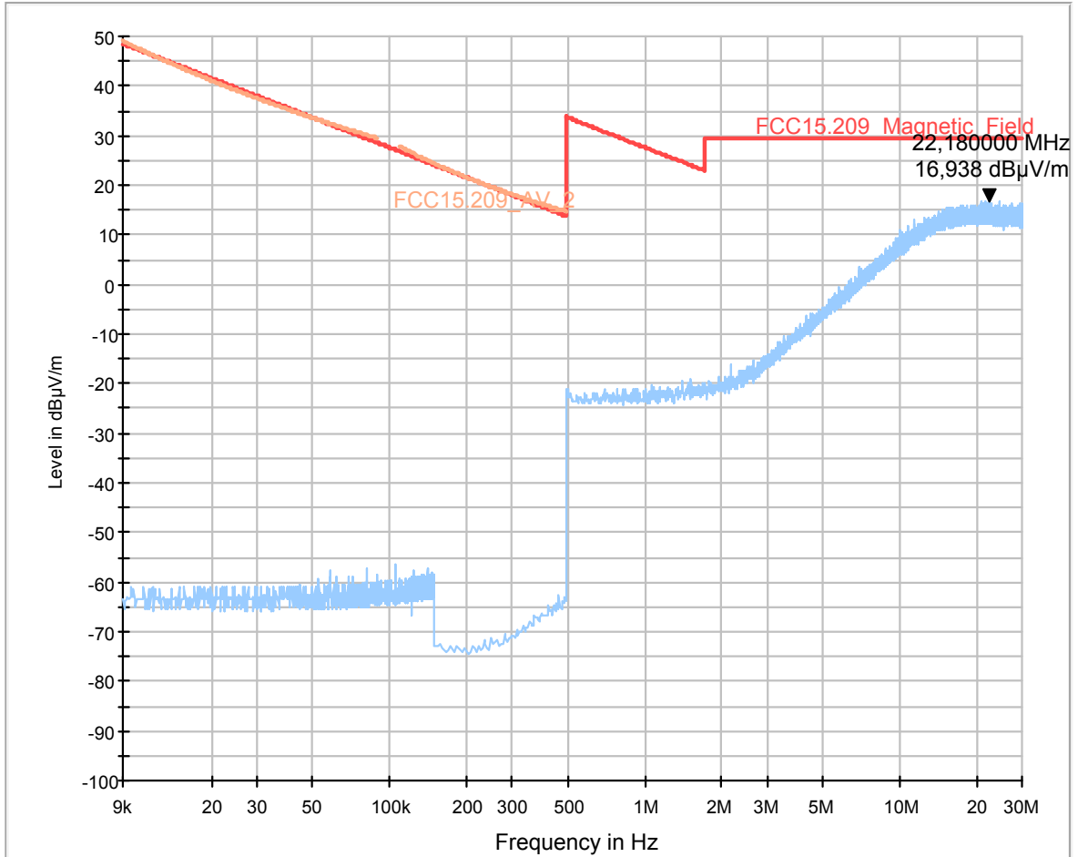
FCC15.209_magn hor+vert
