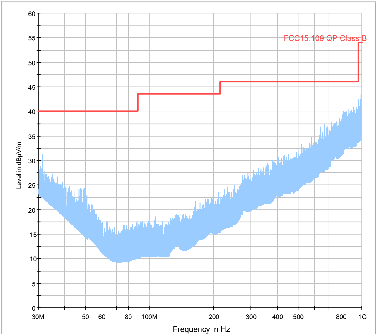
FCC15.109_hor+vert
