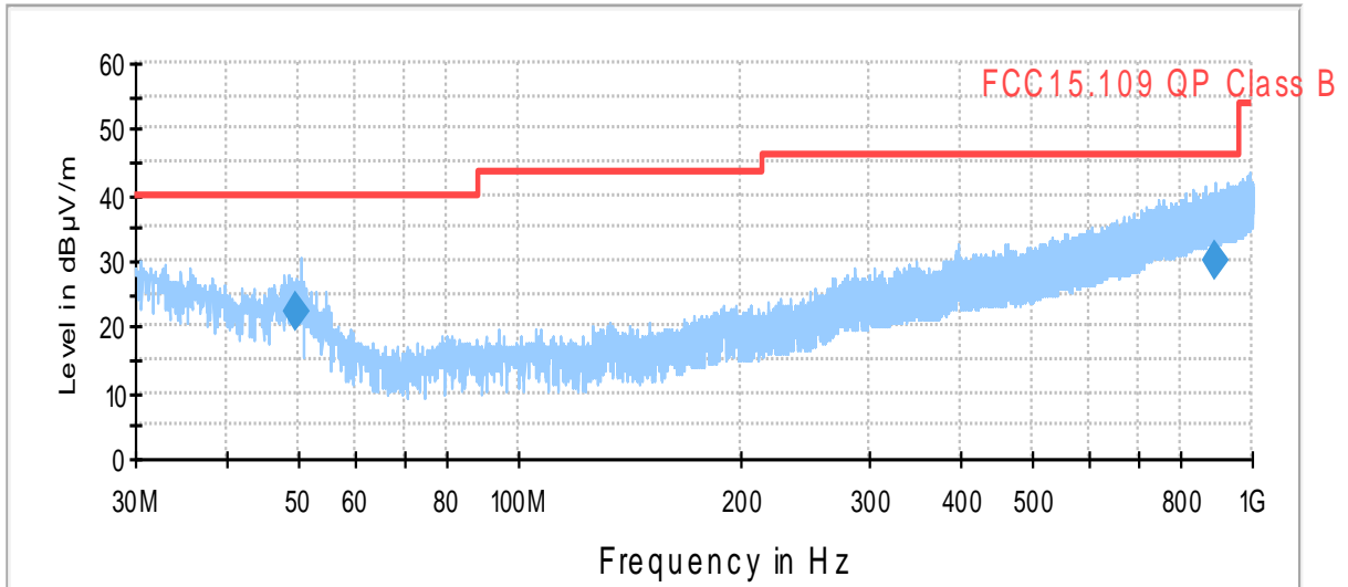
05_FCC15.109_hor+vert_kipp
