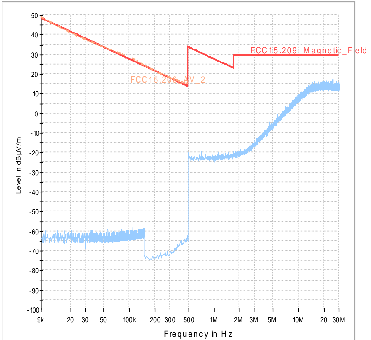
FCC15.209_magn hor+vert
