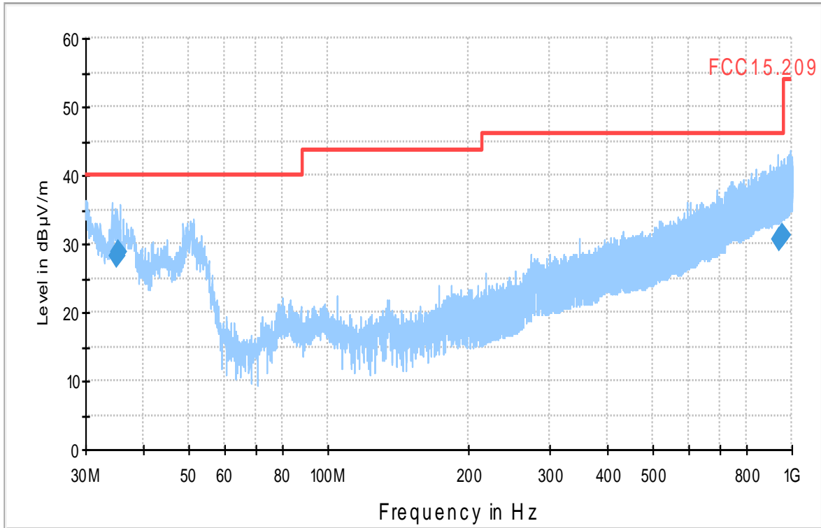
01_FCC15.209_hor+vert_kipp
