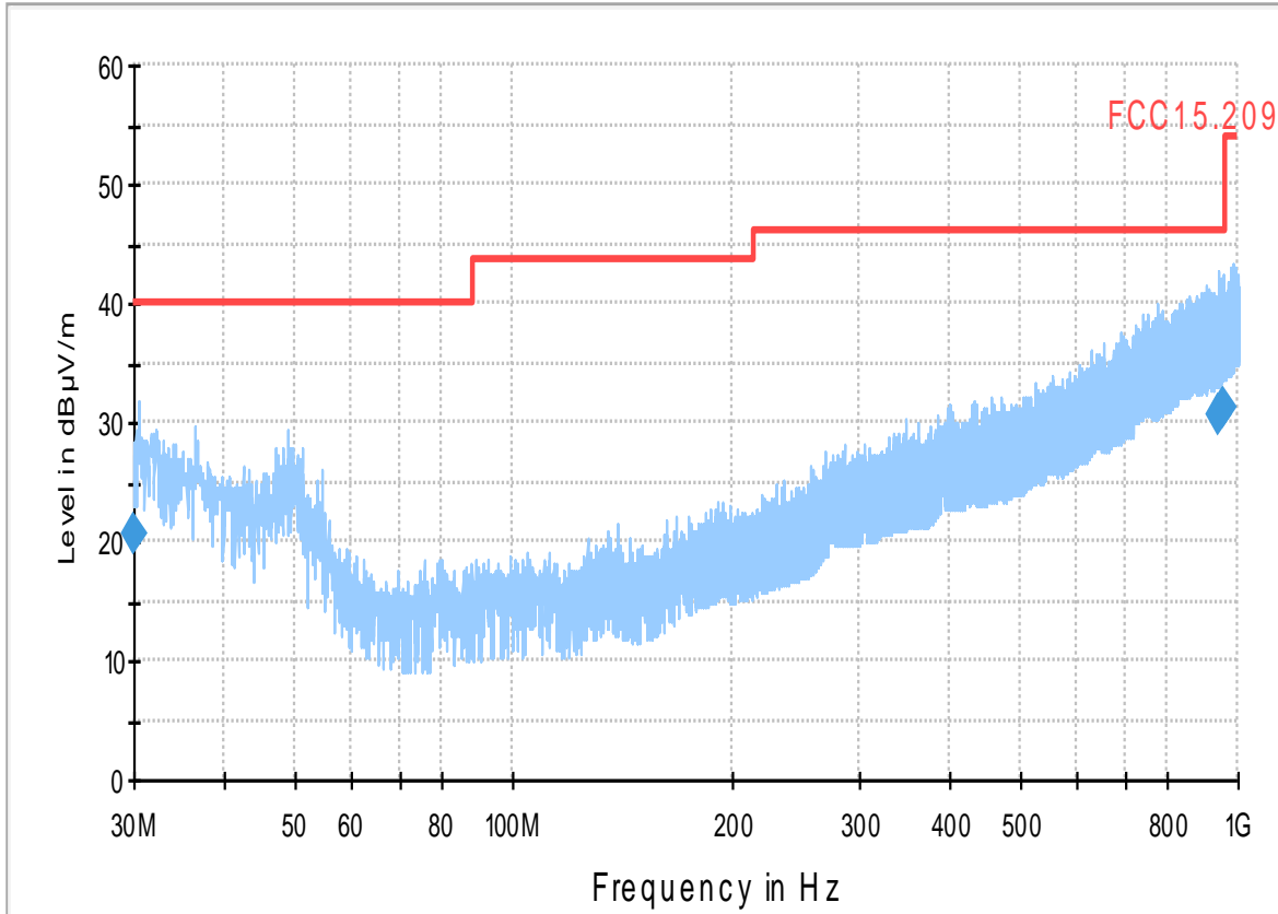
01_FCC15.209_hor+vert_kipp
