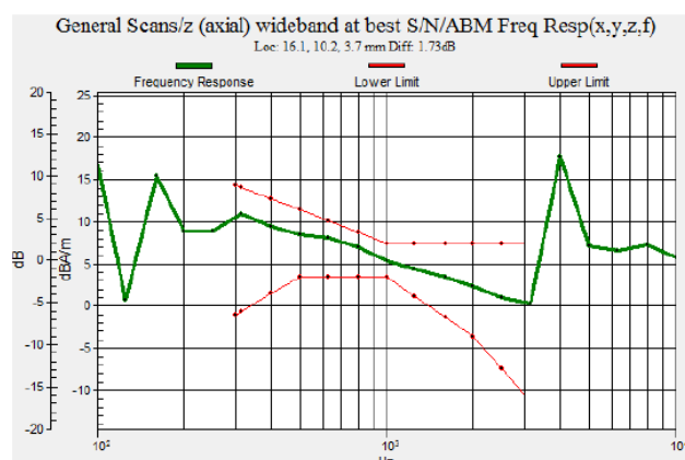
Fig. 7.10 WCDMA Band VI Ch1413
