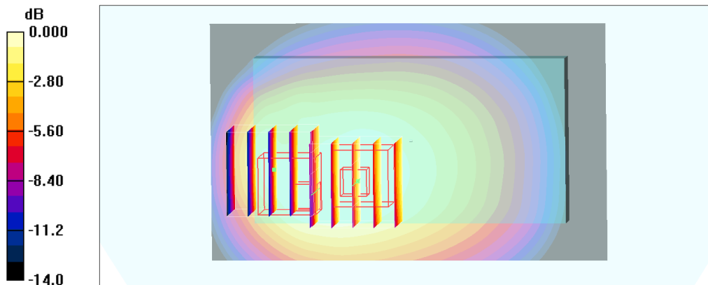
0 dB = 1.40mW/g
