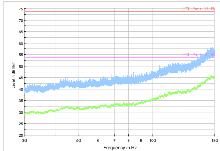
RE - 3GHz-18GHz
