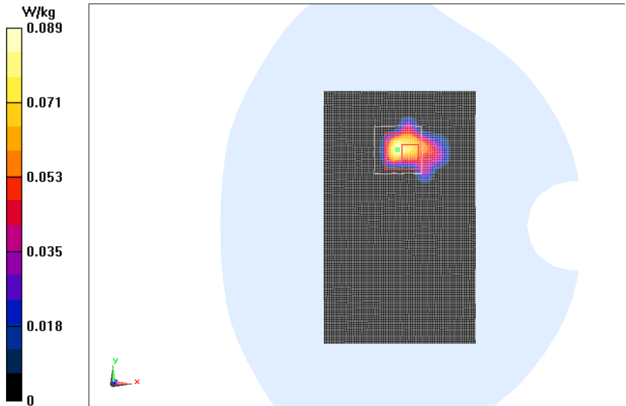
Fig.14 5GHz CH36
