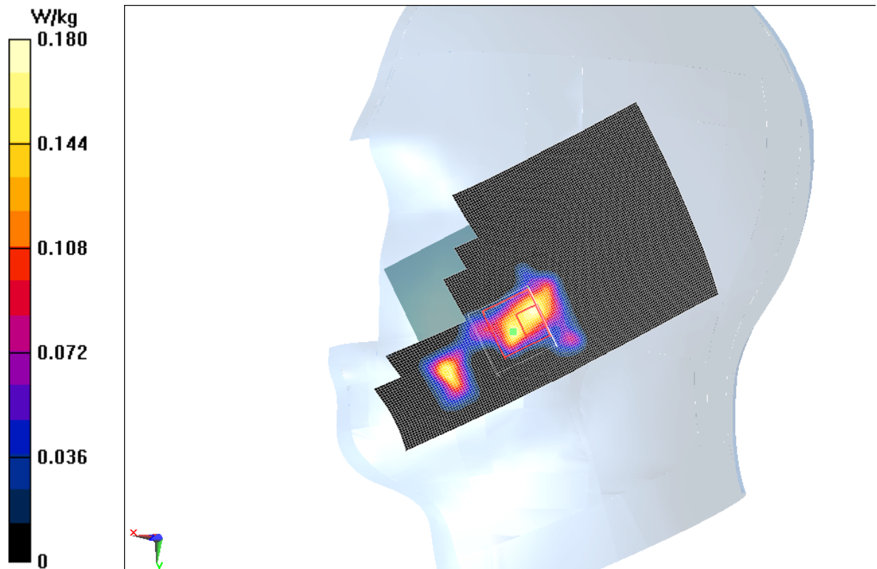
Fig.9 5GHz CH36
