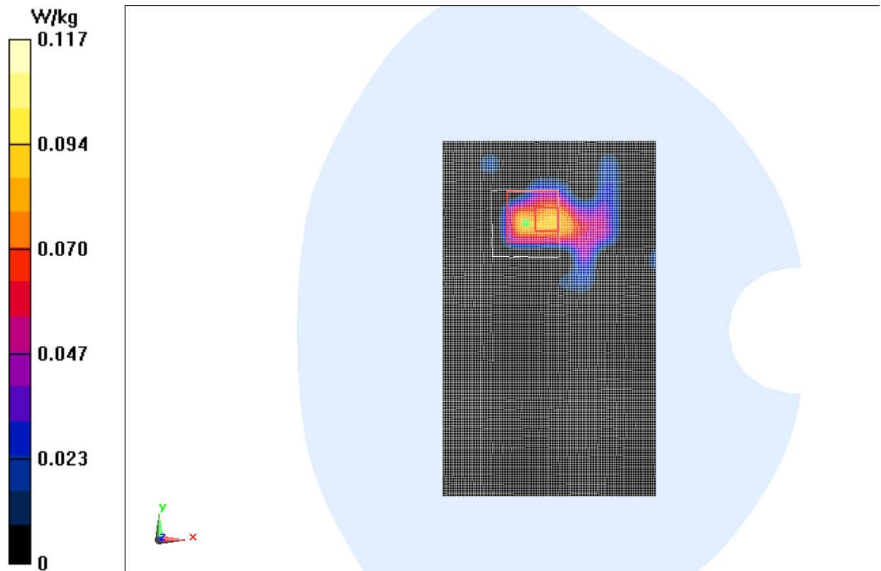
Fig.10 5GHz CH36
