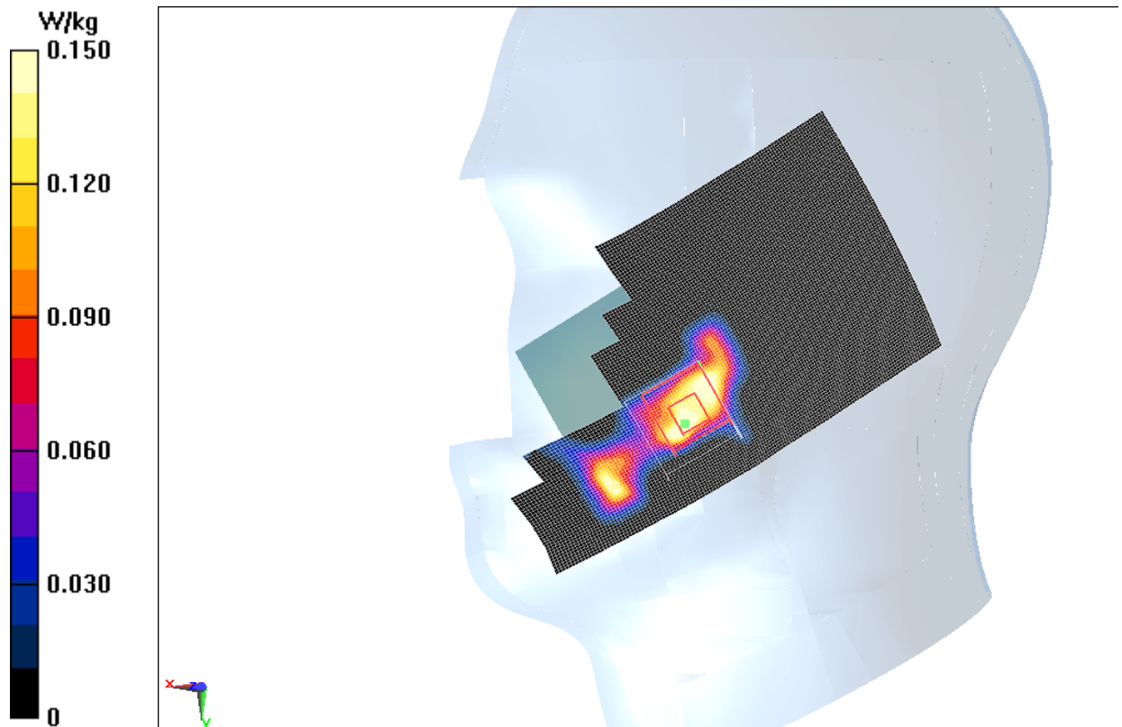
Fig.13 5GHz CH36
