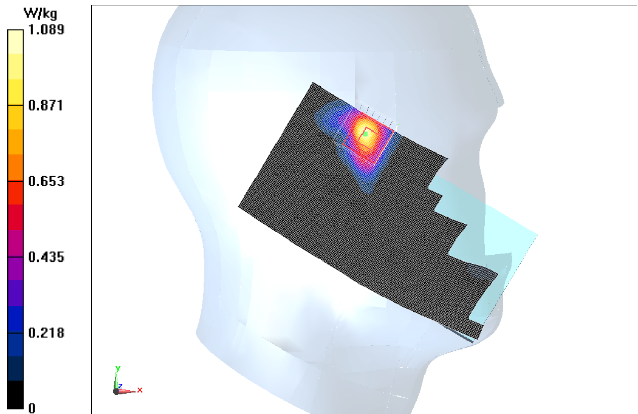
Fig.31 5GHz CH42
