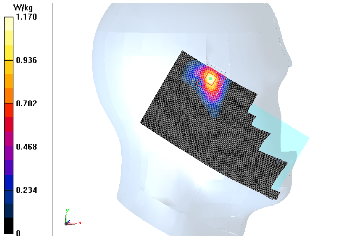
Fig.27 5GHz CH60
