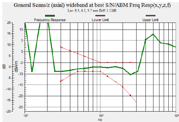
Fig 7.1 GSM850 Ch189
