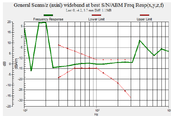
Fig 7.3 GSM850 Ch4182
