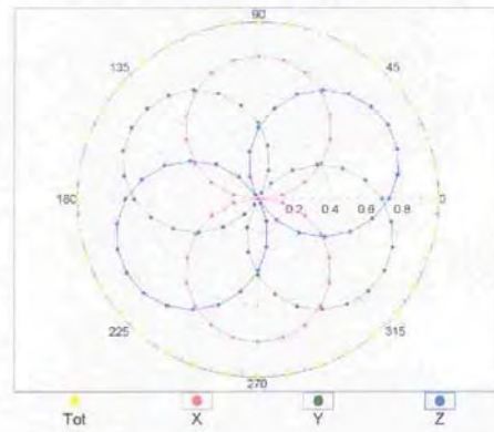
f=1800 MHz,R22
