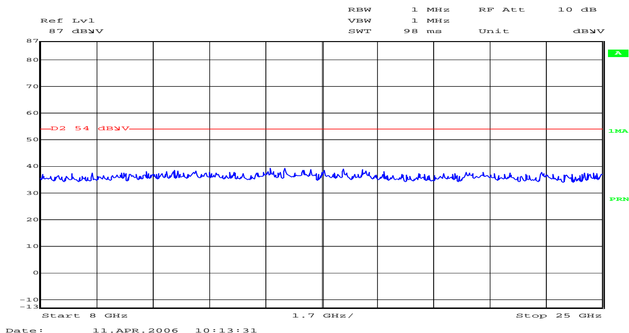
Plot 11 of 11: RX Mode ( 8GHz – 25GHz)
