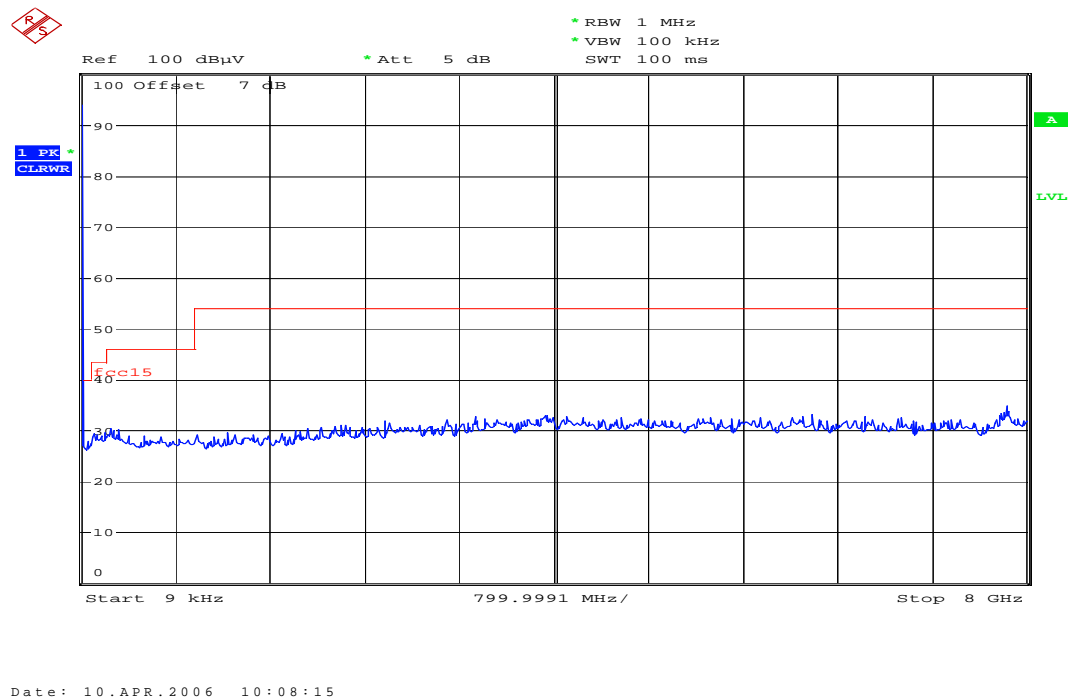
Plot 10 of 11: RX Mode( 9kHz – 8GHz)
