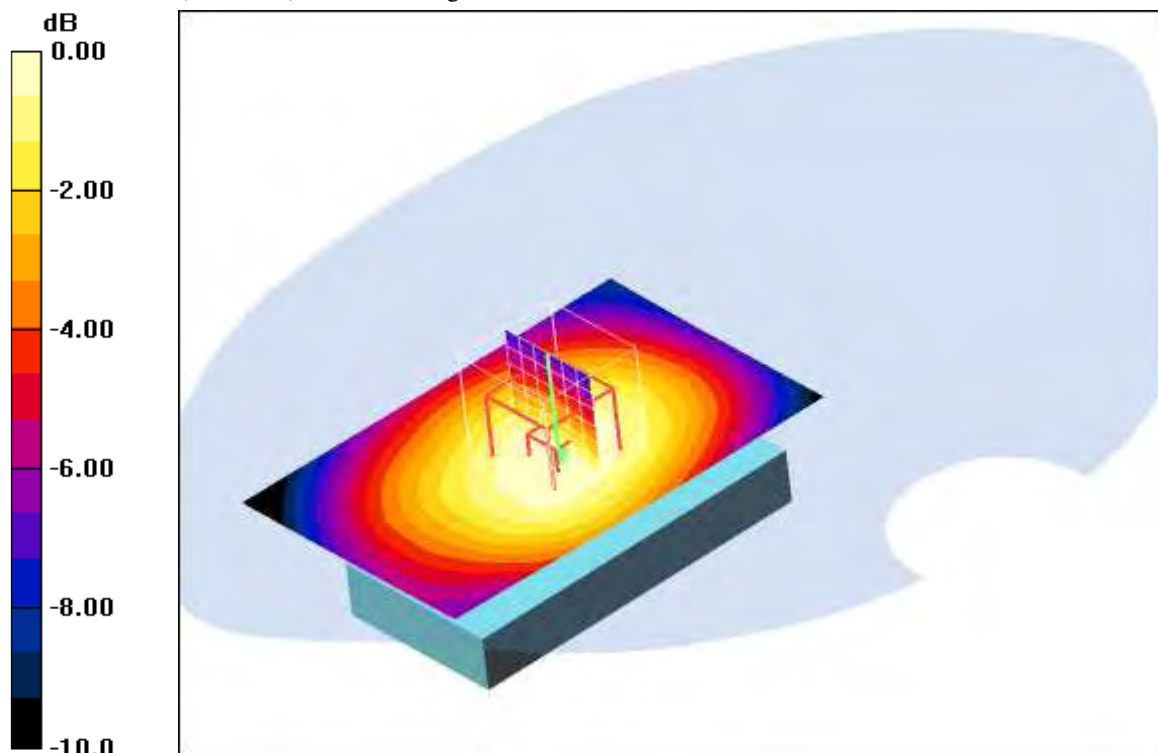
0 dB = 0.171mW/g
