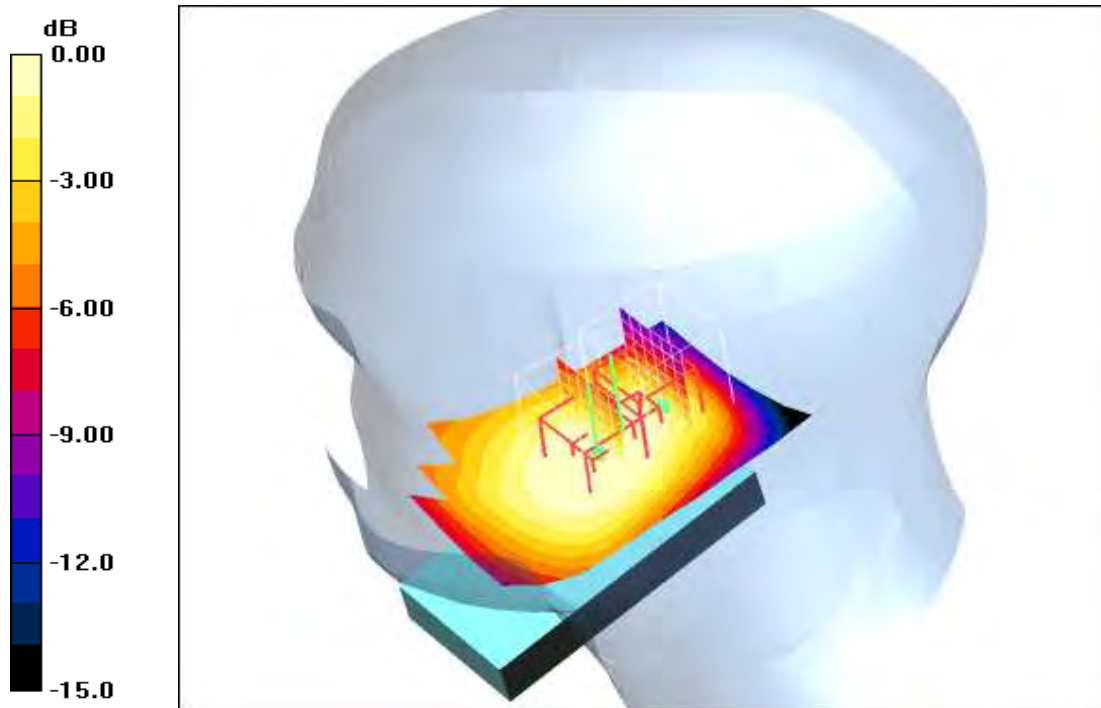
0 dB = 0.193mW/g
