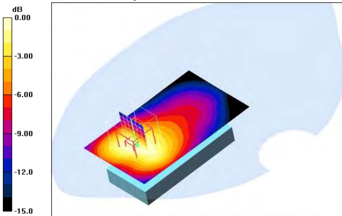
0 dB = 0.192mW/g
