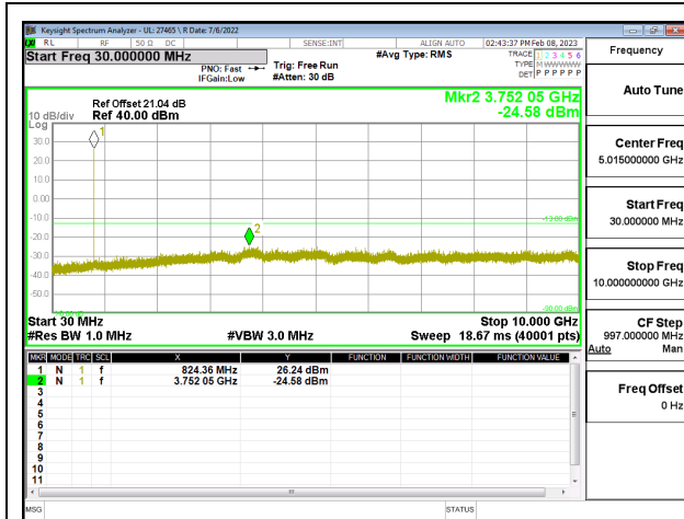
5G NR n5 5MHz QPSK LOW Ch RB1-0
