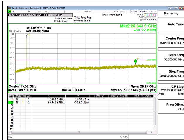
5G NR n41 40MHz BPSK LOW Ch RB1-0
