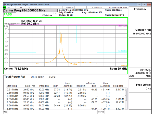
LTE13 5MHz QPSK HIGH Ch RB1-0
