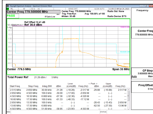
LTE13 5MHz 16QAM LOW Ch RB25-0
