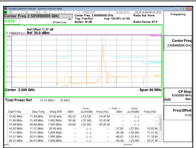
5G NR n41 20MHz 16QAM Low Channel RB1-49
