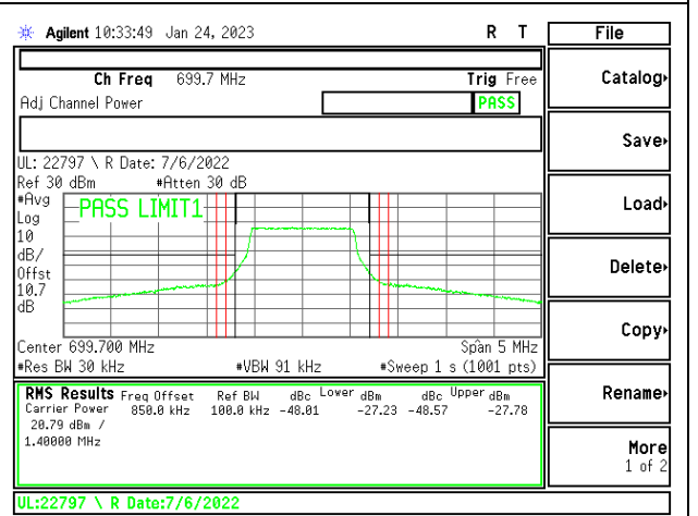
LTE12 1.4MHz QPSK HIGH Ch RB6-0
