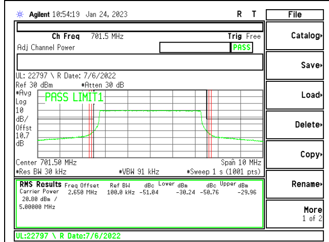
LTE12 5MHz QPSK LOW Ch RB25-0
