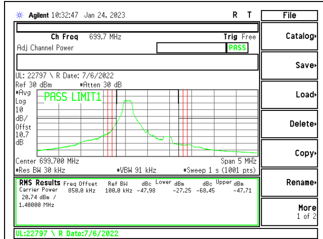
LTE12 1.4MHz QPSK LOW Ch RB1-0
