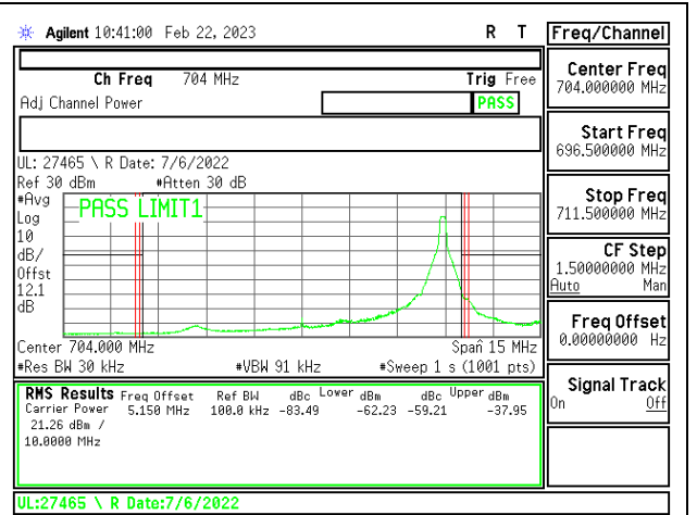
LTE12 10MHz QPSK LOW Ch RB1-49
