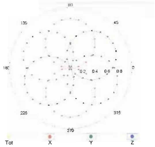
f=1800 MHz,R22
