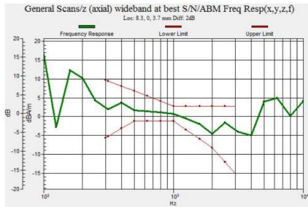
Fig 7.3 WCDMA V Ch4182
