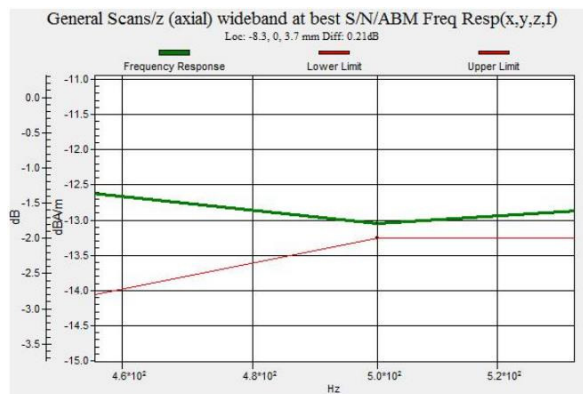
Fig 7.1 GSM850 CH 189
