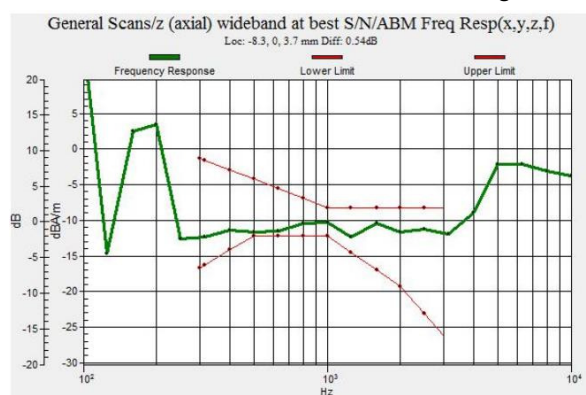
Fig 7.2 GSM1900 CH 661
