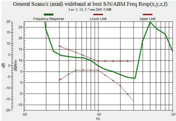
Fig 7.1 GSM850 Ch189
