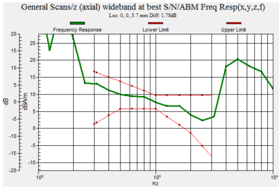
Fig 7.1 GSM850 Ch189
