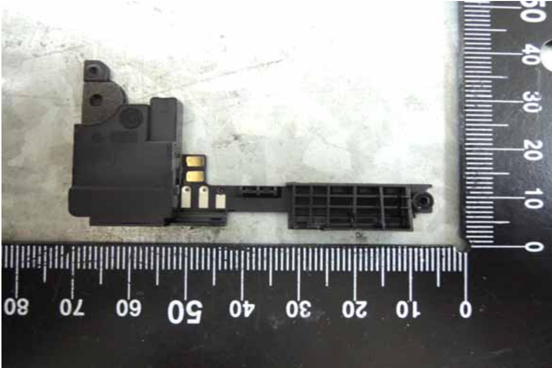
WWAN Antenna (Aux) - 1
