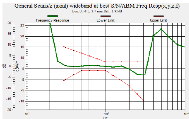
Fig 7.1 GSM850 Ch189
