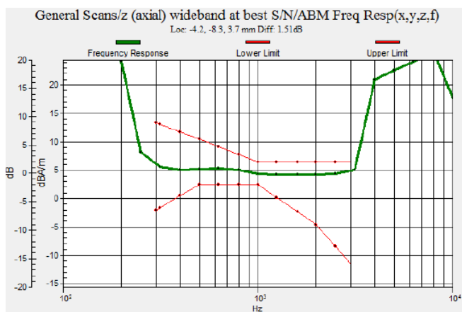
Fig 7.1 GSM850 Ch189
