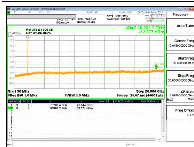
5G NR N66 20MHz QPSK MID Ch RB1-0
