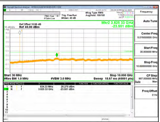
5G NR n5 5MHz QPSK MID Ch RB1-0
