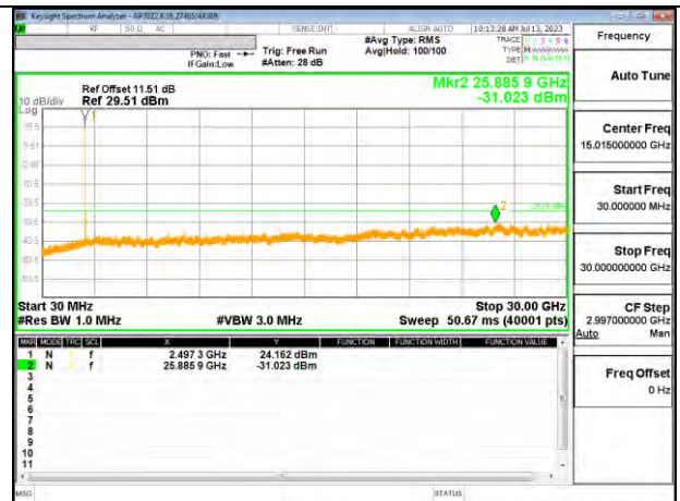
5G NR n41 30MHz QPSK LOW Ch RB1-0
