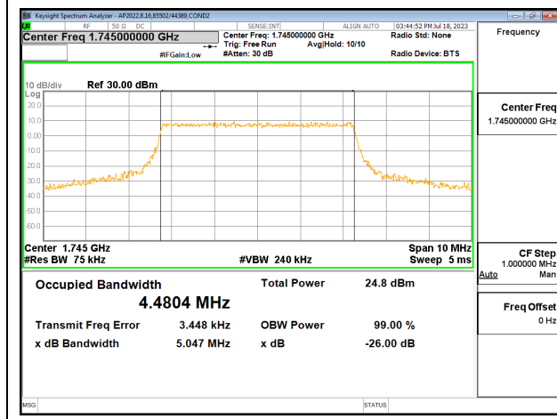
LTE66 5MHz QPSK MID Ch RB25-0
