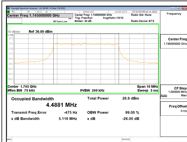
5G NR N66 5MHz QPSK MID Ch RB25-0
