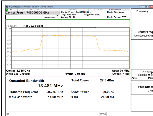
5G NR N66 15MHz QPSK MID Ch RB75-0
